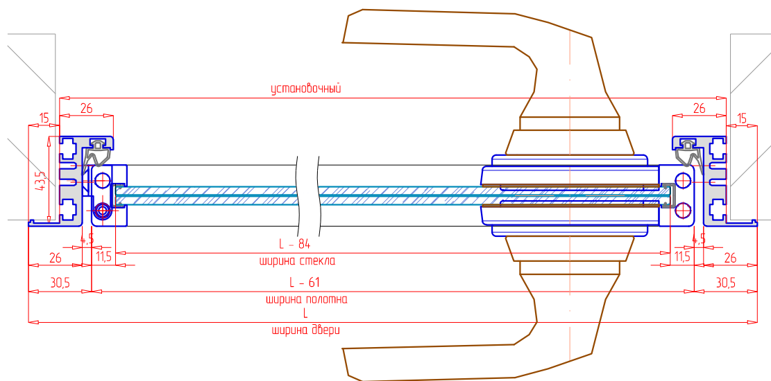
горизонтальное сечение (с круглой накладкой)
