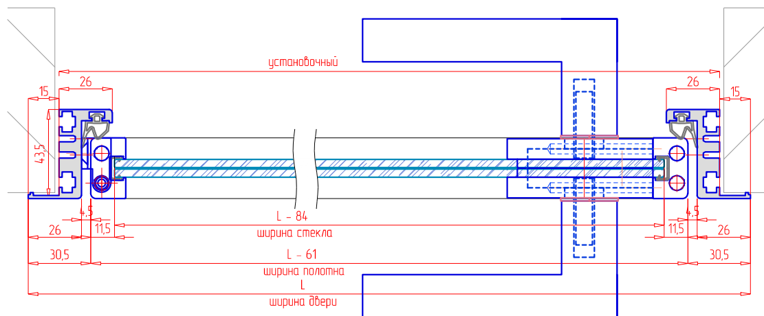
горизонтальное сечение (с прямоугольной накладкой)
