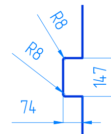
вырез в стекле под круглую накладку
