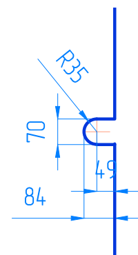
вырез в стекле под круглую накладку
