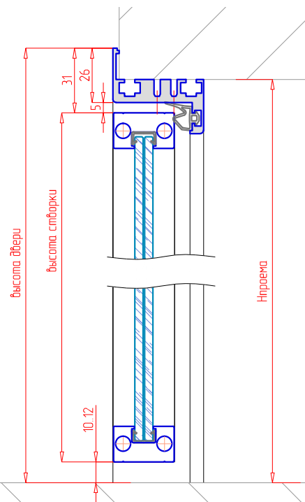
вертикальное сечение
